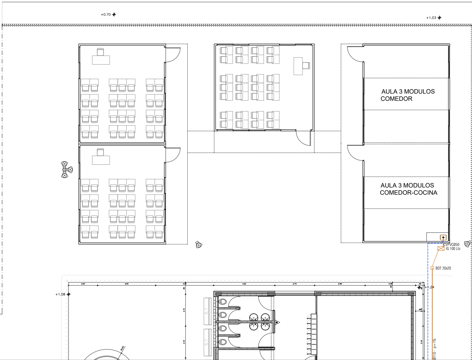
PLANTA AULAS Esc. 1:150
