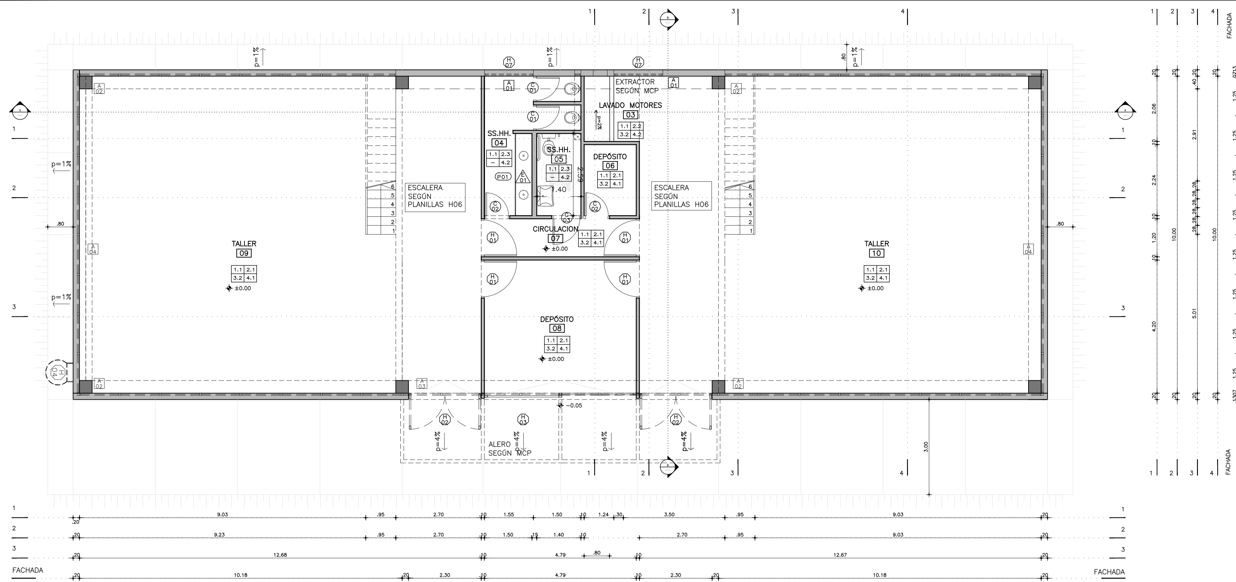
PLANTA NIVEL ± 0.00 Esc 1.75
