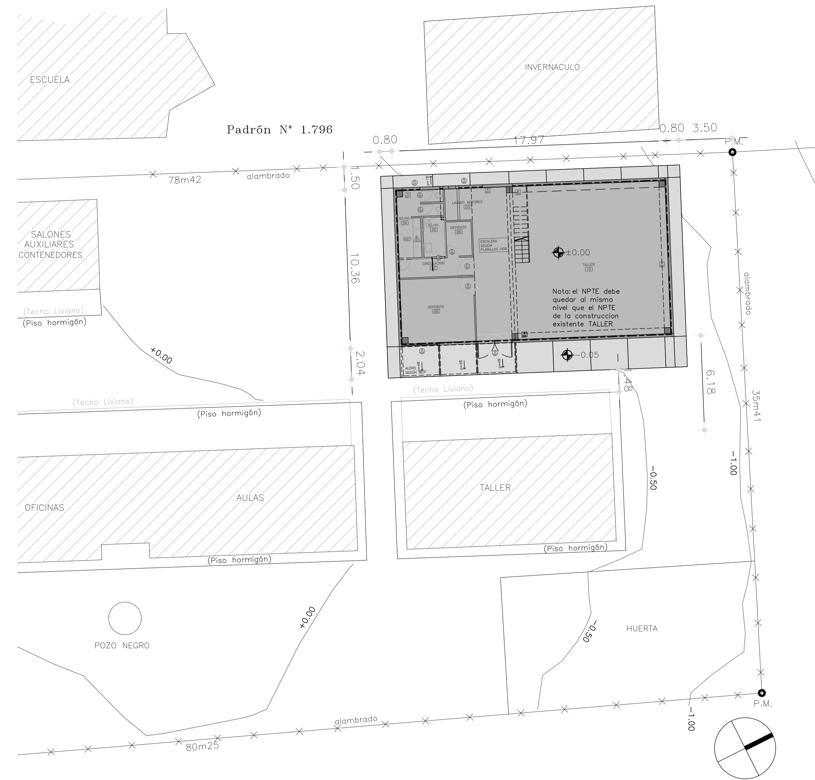
IMPLANTACIÓN ESCALA 1:200
